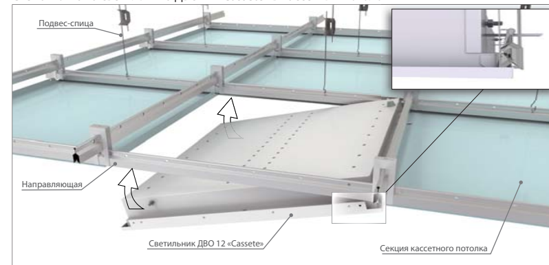
Схема монтажа светильника ДВО 12 «Cassete» в кассетный потолок
